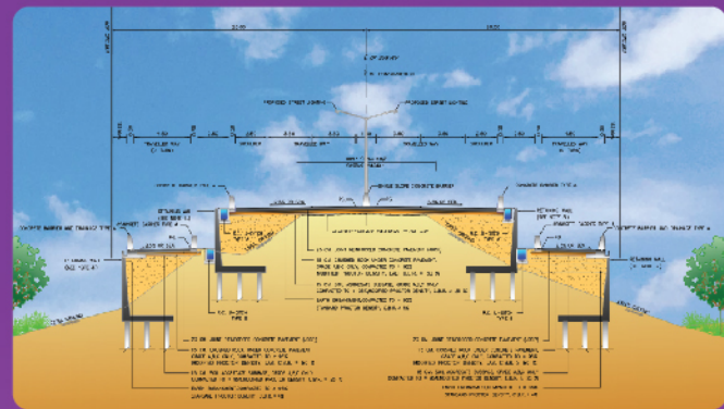
กำแพงกันดินมีเสาเข็ม บริเวณจุดกลับรถได้สะพาน
