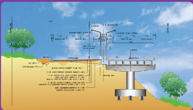
รูปแบบโครงสร้างสะพาน ในกรณีก่อสร้างด้านใดด้านหนึ่ง
