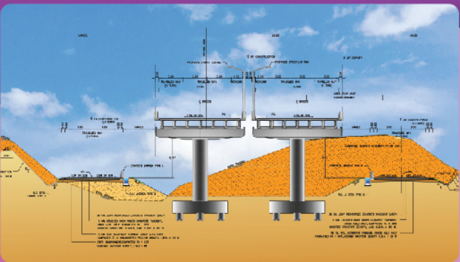
รูปแบบโครงสร้างสะพาน บริเวณ กม.24+088 กลับรถได้สะพานได้ 2 ทิศทาง
