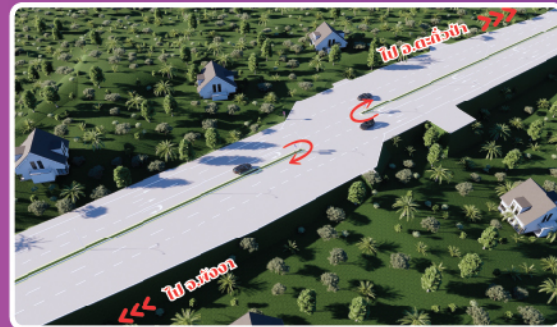
แสดงจุดกลับรถระดับพื้น บริเวณ กม.25+882 (กลับรถได้ 2 ทิศทาง)
