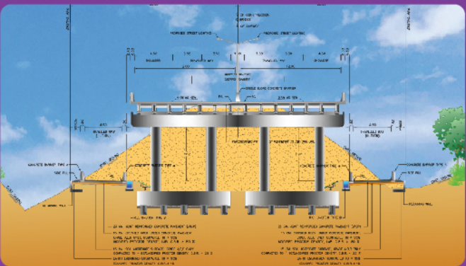
รูปแบบโครงสร้างสะพานบริเวณ กม.21+730 กลับรถได้สะพานได้ 1 ทิศทาง
