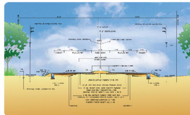
ช่วงที่ผ่านพื้นที่ทางลาดชันน้อย (ช่วงผ่านพื้นที่ชุมชน)
